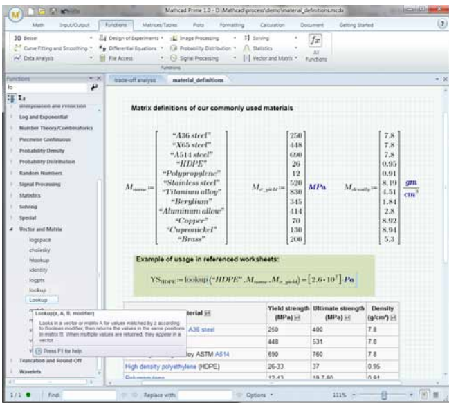
Abbildung E: Mathcad Tabelle mit Streckfestigkeit, Zugfestigkeit und Dichte unterschiedlicher Materialien
