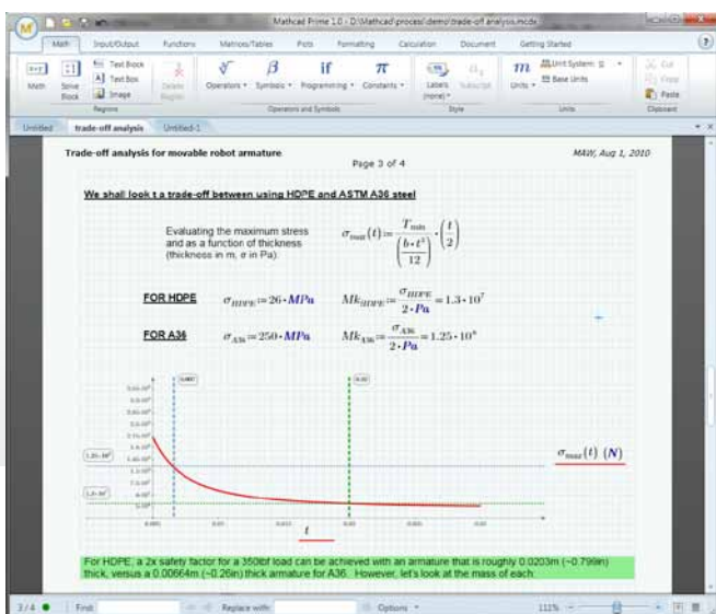
Abbildung F: Diagramm der Tradeoff-Analyse zwischen Polyethylen-HDPE und ASTM A36-Stahl
