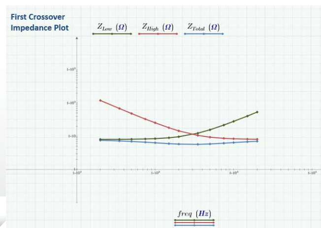
Abbildung D: Mathcad Übergangs-Plot der Impedanz-Tradeoffs erster Ordnung
